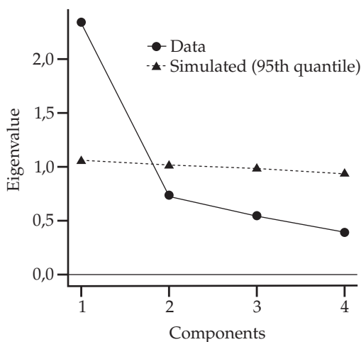
Obrázek 3. Paralelní analýza
